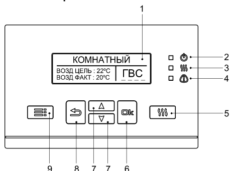
Рисунок 2. Блок управления
